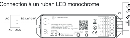
Connection à un ruban LED monochrome
