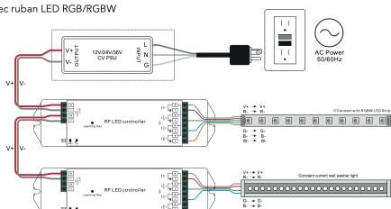
Avec ruban LED monochrome
